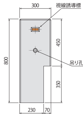
側面図
