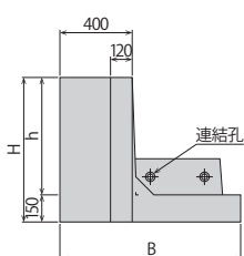
側面図
