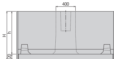
背面図
