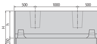
背面図
