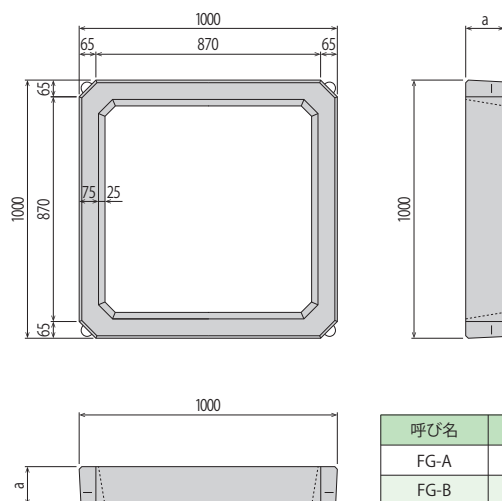
製品図
