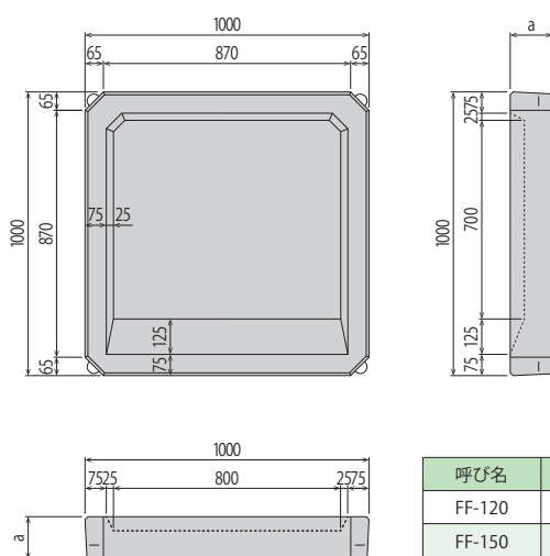
製品図
